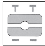
Schlepprossenschuh zweiteilig, Anbringung nach Konfektionierung Type Standard d 44 bis 76mm Type Extra Heavy Duty Plus d 60 bis 90mm
